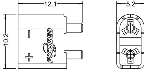
安装堆叠尺寸 (mm)
