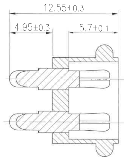
A-A' 剖面图
