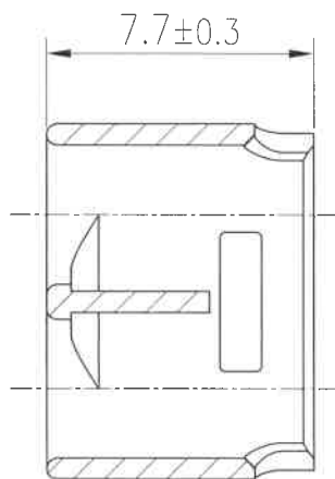
A-A' 剖面图
