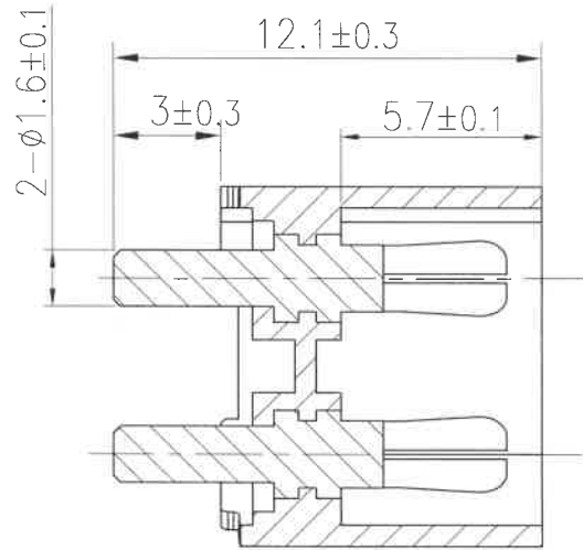
A-A' 剖面图
