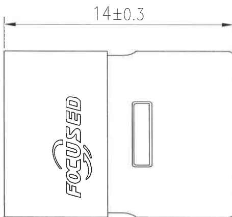
FCB20-M含后盖尺寸
