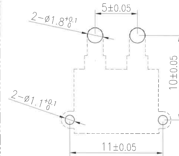
板端布板尺寸
