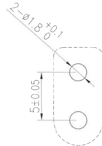
板端布板尺寸
