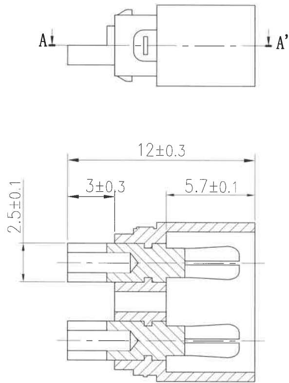
A-A' 剖面图
