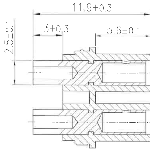
A-A' 剖面图
