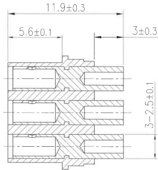
A-A' 剖面图
