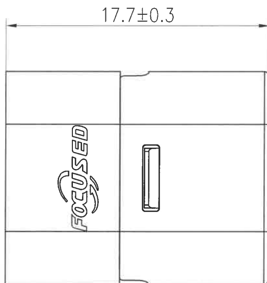
FCB40-M含后盖尺寸
