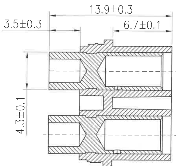
A-A' 剖面图
