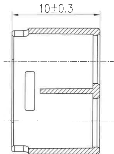
A-A' 剖面图
