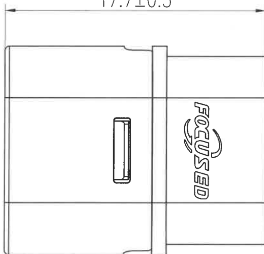
FCB40-F含后盖尺寸
